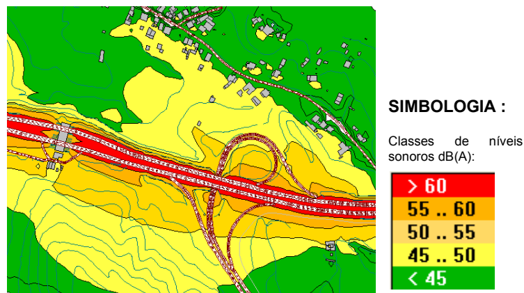
Figura 3 – Exemplo de um mapa de níveis sonoros, para o Indicador de Ruído L_n
